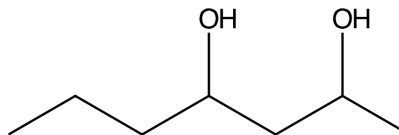
2,4-Heptanediol
