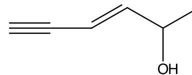
trans -3-Hexen-5-yn-2-ol
